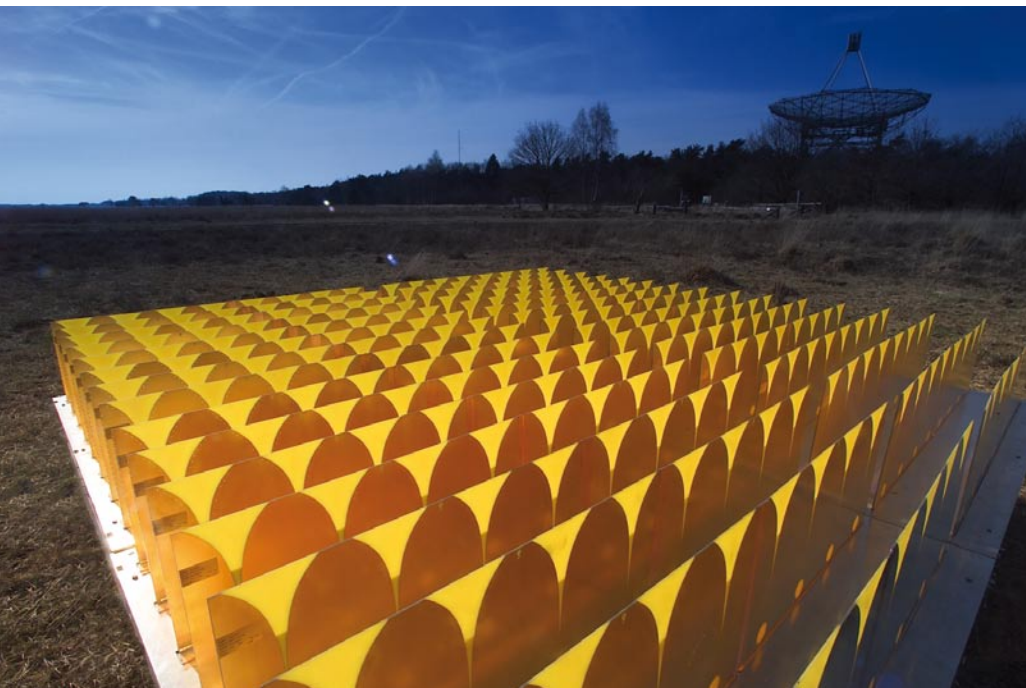
▼ Abb. 6: Ein Prototyp aus Halbleiter-»Kacheln« zur Messung von Radiowellen bei Frequenzen um 1 GHz ist das Thousand Element Array (TEA). (Quelle: ASTRON)
